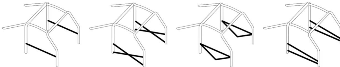
شکل ۳: روش های مجاز نصب رول بارهای سقفی
