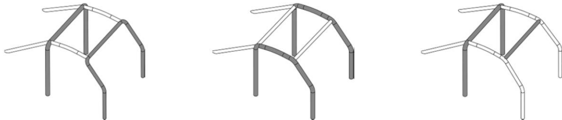
شکل ۳: روش های مجاز نصب رول های کناری
