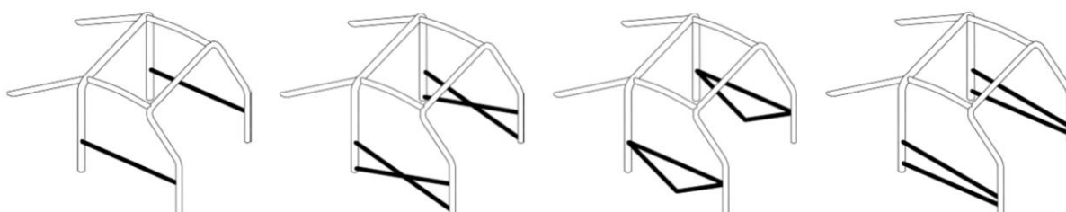
شکل ۴: روش های مجاز نصب رول بارهای سقفی
